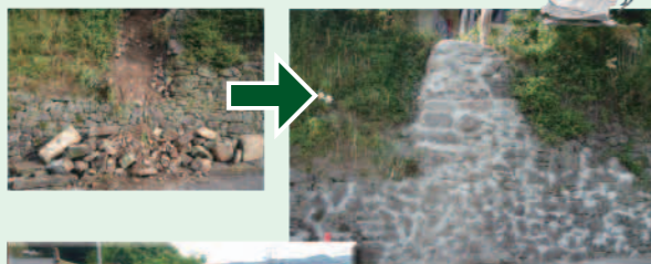
市道への落石対策
